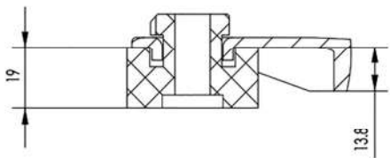
A-A 1:2
