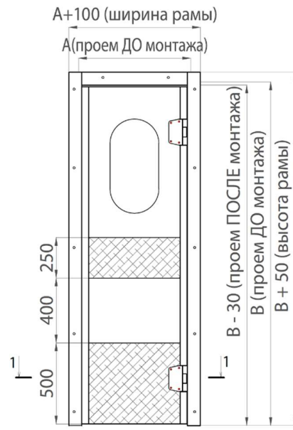
Рисунок 79. МДО с угловой рамой
