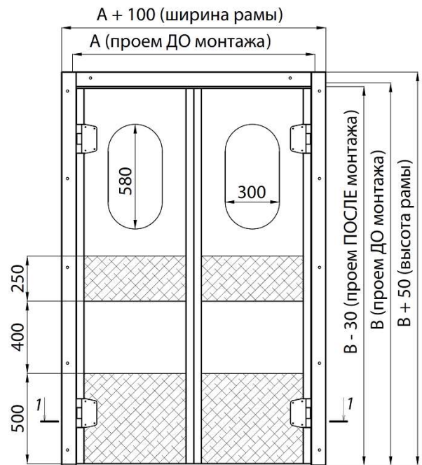
Рисунок 105. МДД с рамой, устанавливаемой в обхват проема
