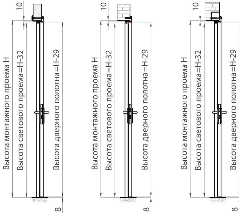
Крепление к панели Крепление к кирпичной стене Крепление к металлоконструкции
