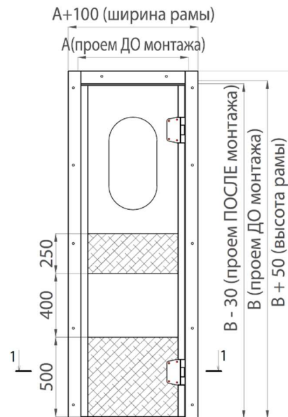
Рисунок 88. МДО с металлической рамой, устанавливаемой в обхват проема
