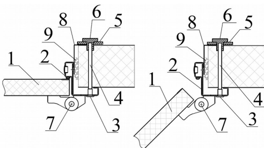
Рисунок 123. Разрез 4-4. ТДО с угловой рамой с порогом 60 мм
