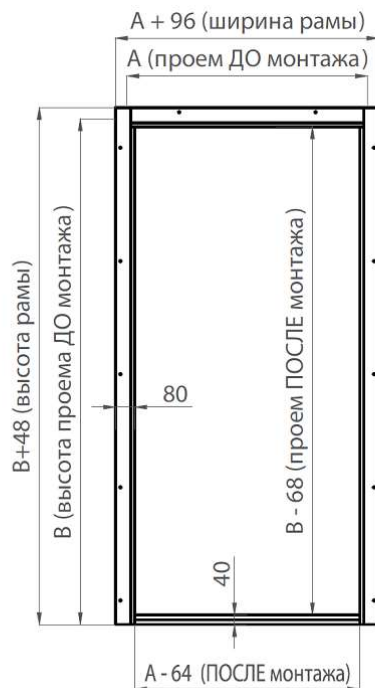
Рисунок 128. Металлическая рама с порогом 40 мм, устанавливаемая в обхват проема
