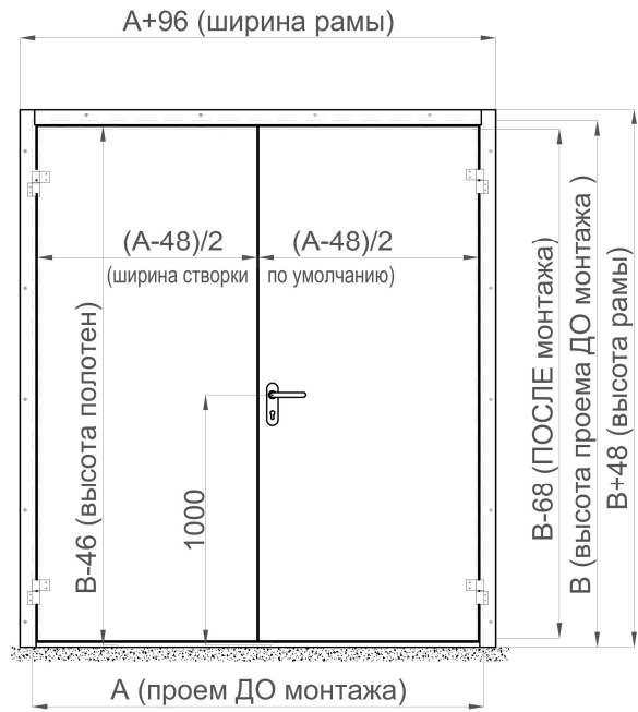
Рисунок 143. ТДД с угловой рамой с порогом 40 мм
