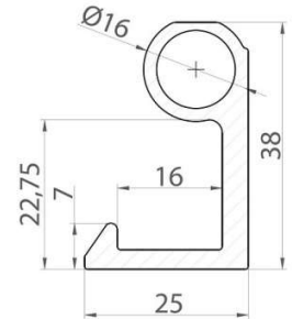
Рисунок 4. Профиль уплотнительный нижний
