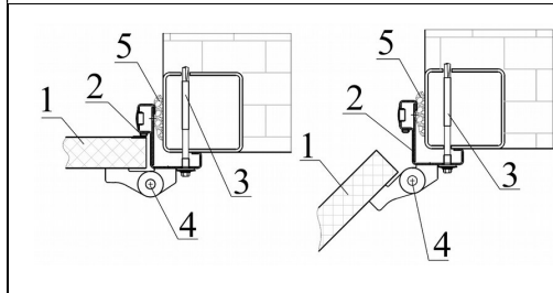
Рисунок 156. Узлы крепления металлической угловой рамы к металлокаркасу (слева — узел 5, справа — узел 6)
