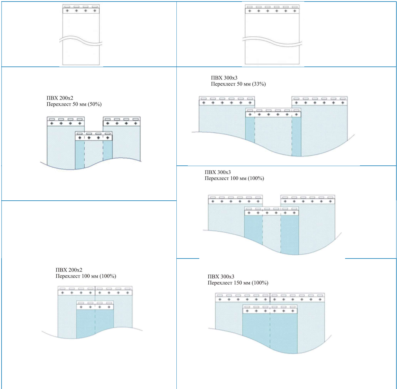
Рисунок 15. ПВХ-ленты шириной 200 и 300 мм с разным перехлестом
