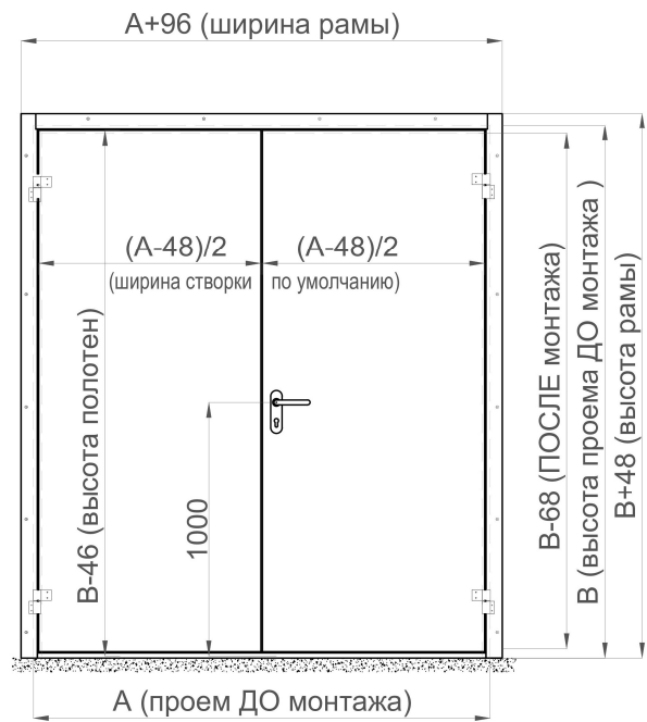
Рисунок 161. ТДД с рамой в обхват проема с порогом 40 мм
