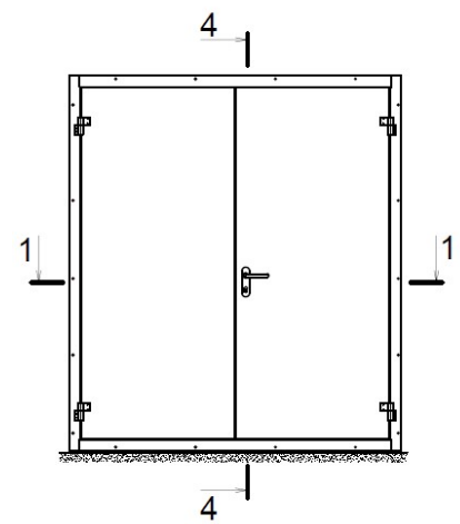
Рисунок 165. Местоположение разрезов на ТДД с порогом 60 мм
