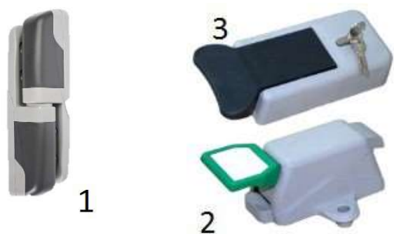
Рисунок 36. Фурнитура РДД: 1 — дверная петля подъемного типа с регулировками в трех плоскостях Fermod, 2 — внутренняя ручка аварийного открывания МТН, 3 — наружная ручка со встроенным замком МТН
