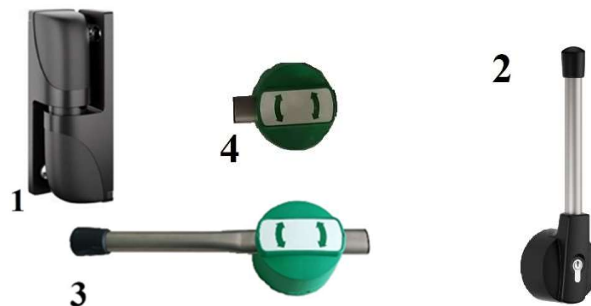
Рисунок 37. Фурнитура РДД серии S (Stuv): 1 — дверная металлическая петля с регулировками в трех плоскостях, 2 — наружная поворотная ручка со встроенным замком, 3 — внутренняя поворотная ручка аварийного открывания, 4 — дополнительный затвор для дверей высотой более 2400 мм
