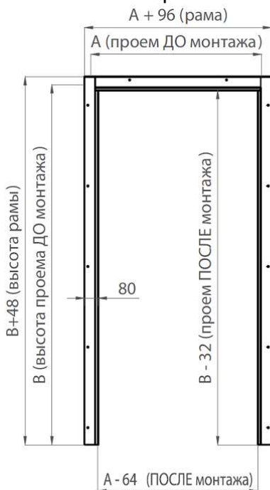
Рисунок 127. Металлическая рама без порога, устанавливаемая в обхват проема
