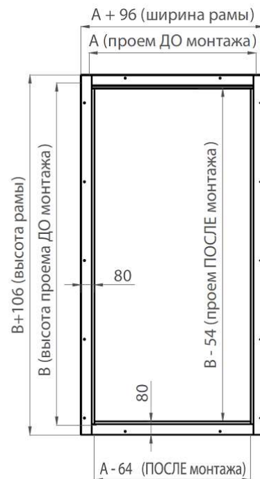
Рисунок 129. Металлическая рама с порогом 60 мм, устанавливаемая в обхват проема
