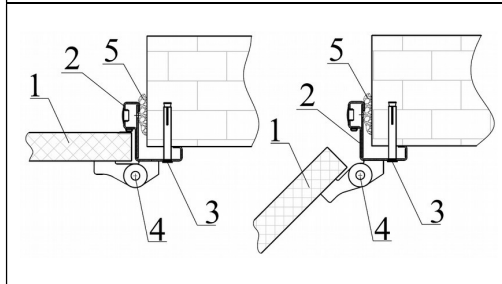
Рисунок 155. Узлы крепления металлической угловой рамы к кирпичной стене (слева — узел 3, справа — узел 4)
