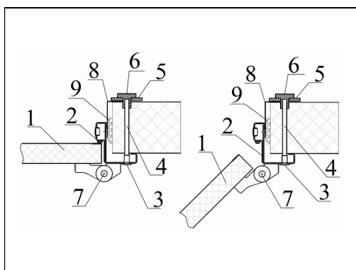
Рисунок 151. Разрез 2-2. ТДД с угловой рамой без порога
