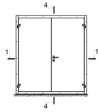
Рисунок 147. Местоположение разрезов на ТДД с порогом 60 мм
