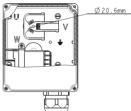
Клеммная коробка
