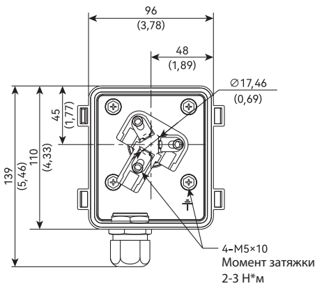
▲ Клеммная коробка
