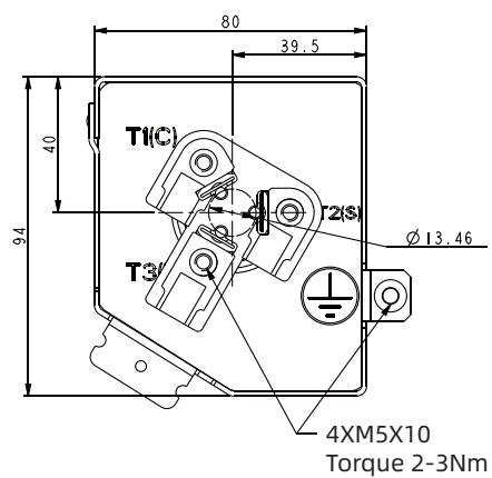
Клеммная коробка
