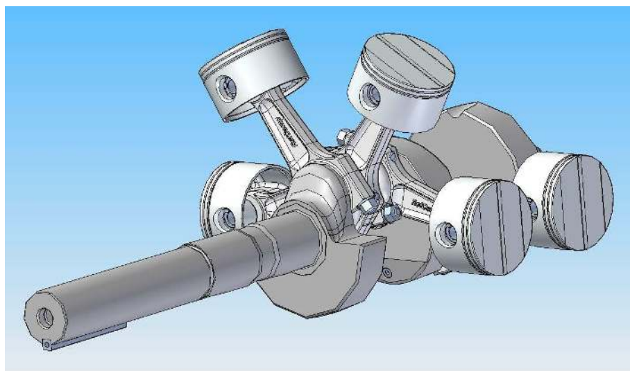
Рисунок 4-6 Вал двигателя и шатун для SP4L1500..2500 SP4H2200..3500 и SP-6 и SP-8
