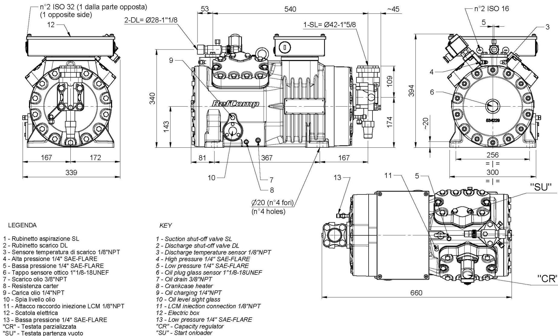
Рисунок 8-6 Габариты моделей SP4HN1500..SP4HN2000
