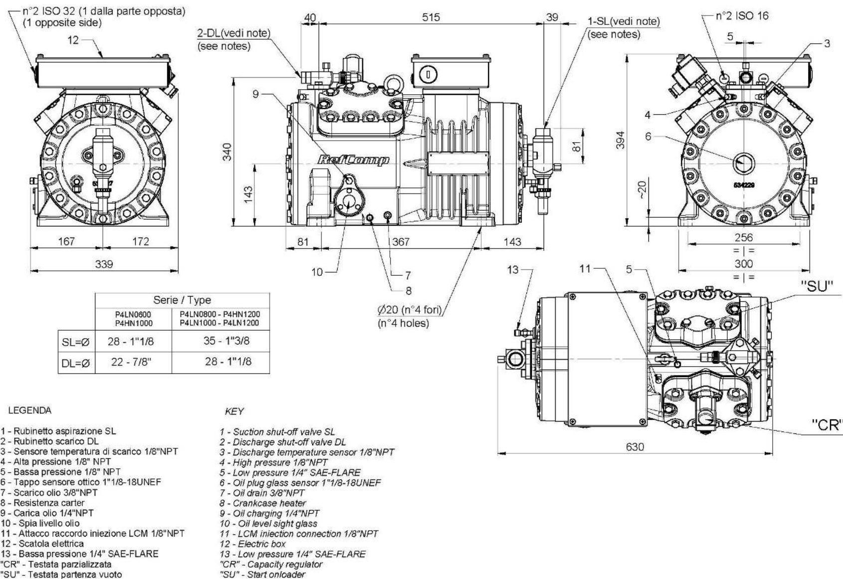
Рисунок 8-5 Габариты моделей SP4LN0600..SP4LN0800 – SP4HN/LN1000..SP4HN/LN1200
