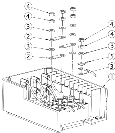
fig.2 / Рис. 2 connection D.O.L. \Delta \Delta - Подключение: O.L.
