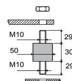
Виброопора
