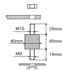
Виброопора
