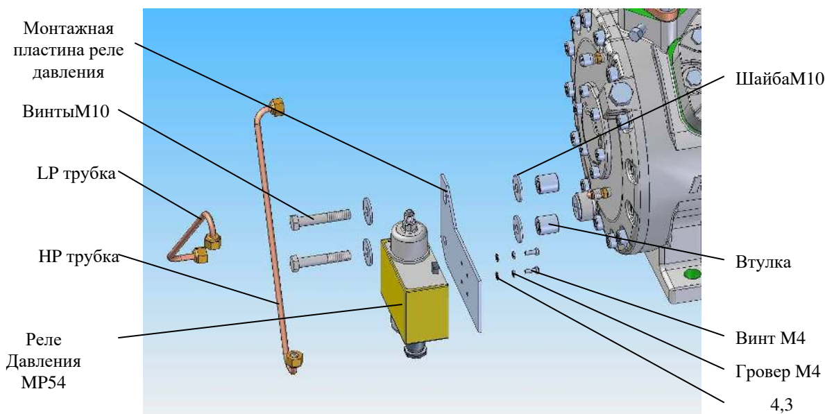
Рисунок 2-22 Компоненты реле давления MP54 для SP4HF 1000-2000 / SP4LF 0600-1200 и SP4HF 100E-200E / SP4LF 060E-120E
