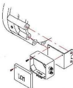
Рисунок 11-5 Сборка электрической коробки LCM
