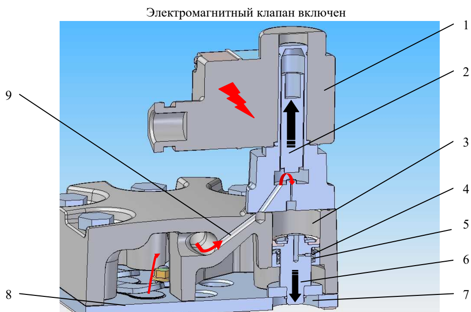
Рисунок 0-1 Принцип работы CR головки
