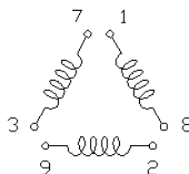
MOTOR WIRINGS
