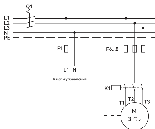
Трёхфазная схема
