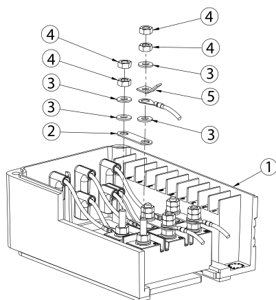
fig.1 / Рис. 1 connection D.O.L. \Delta \Delta - Подключение D.O.L.
