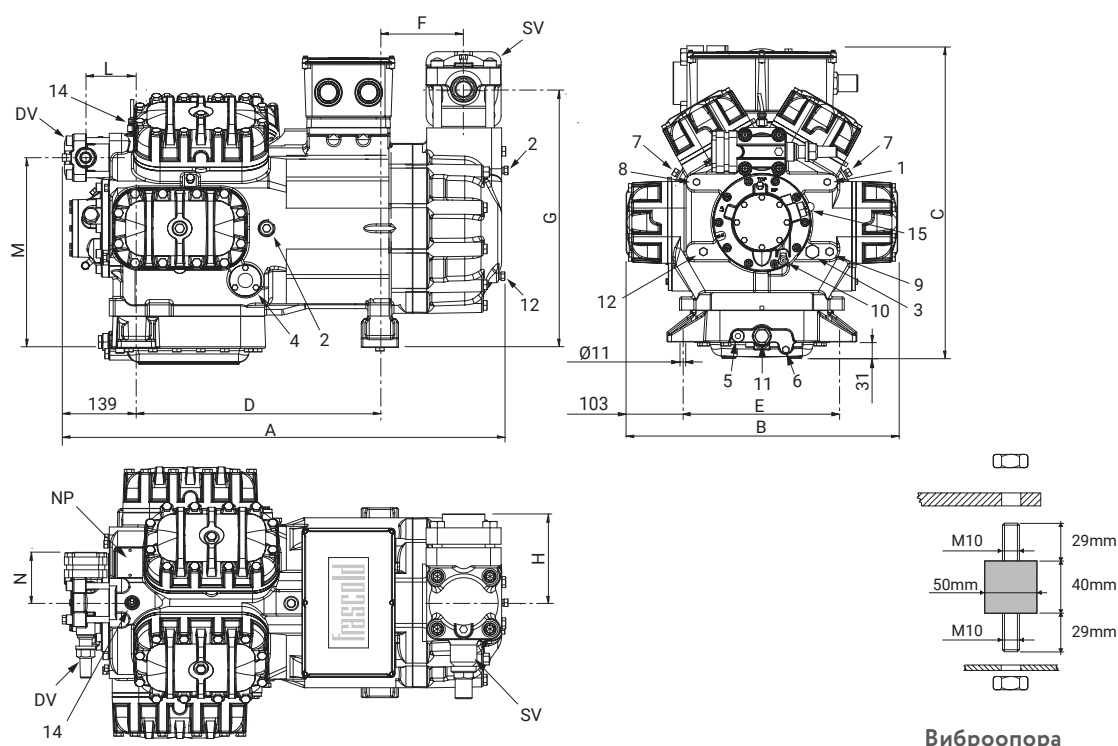
Виброопора
