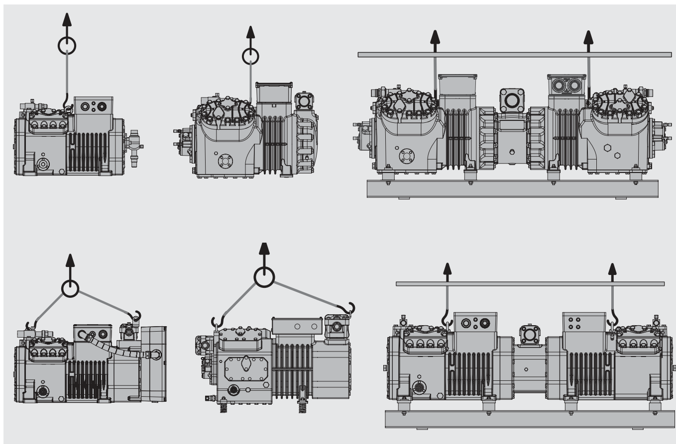
Abb. 1 Verdichter anheben
