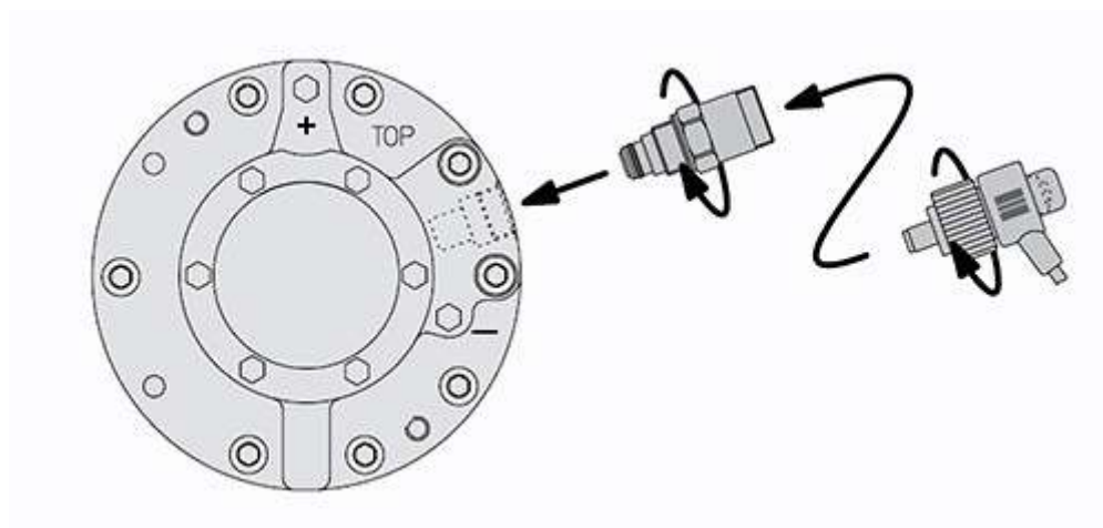
Монтаж Delta-P
