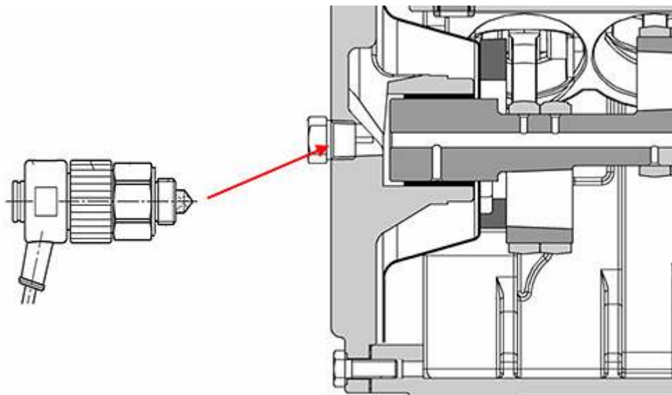
Монтаж OLC-K1
