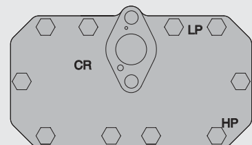
Рис. 3 Головки цилиндров для Р згрузки при пуске / Регулирование производительности
