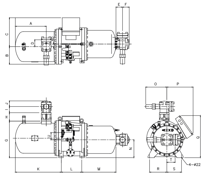
Чертеж RC2-550~RC2-620
