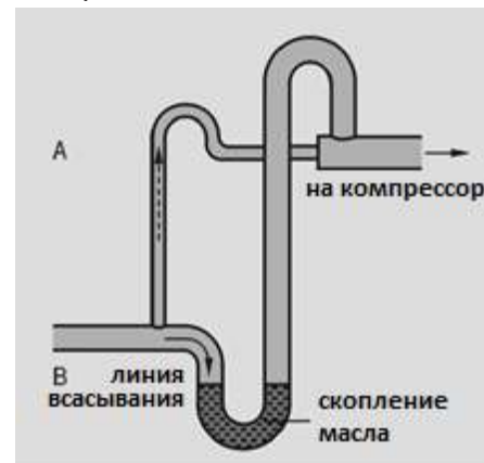
Fig. 11: Вертикальные трубы на стороне всасывания
