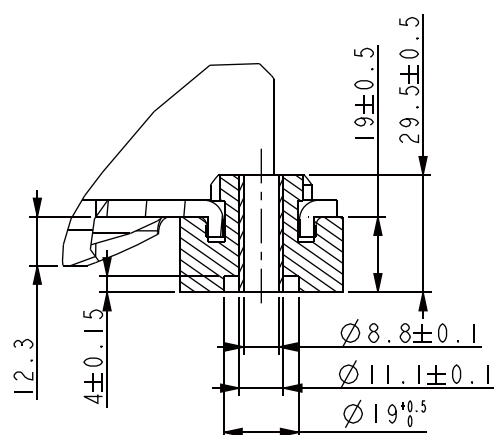
Чертеж виброопоры
