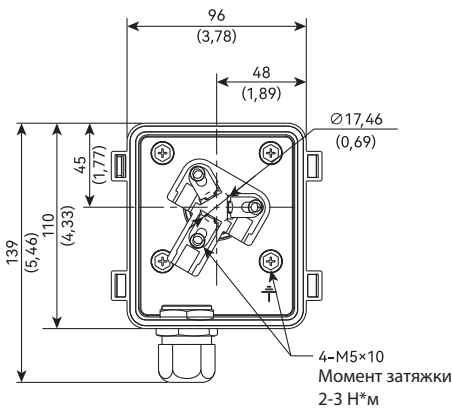
▲ Клеммная коробка
