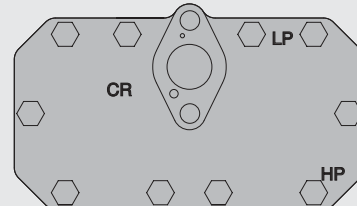
Рис. 3 Головки цилиндров для Разгрузки при пуске / Регулирования производительности
