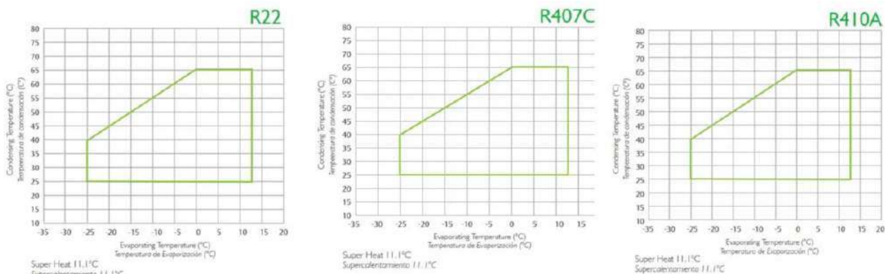
Рис. 2 YH** Область применения для R-22, R-407C и R-410A
