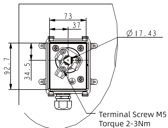
Клеммная коробка
