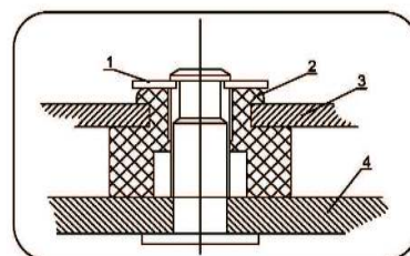
卡簧式 Clamp Type
