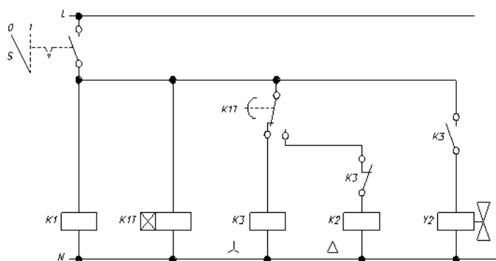
Рисунок 0-8 Звезда-треугольник
