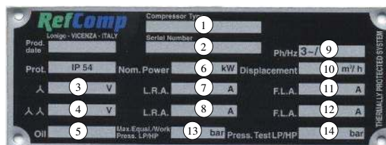
Рисунок 6-1 Заводская табличка для компрессоров с электродвигателем PW и Y/Δ
