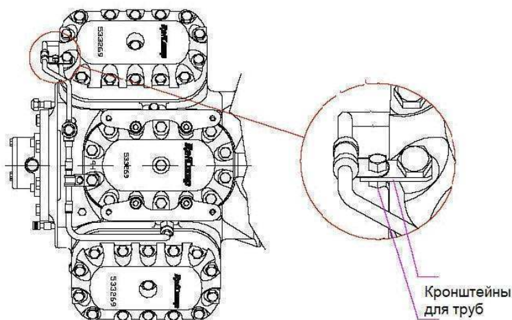
Рисунок 11-4 Кронштейны для труб
