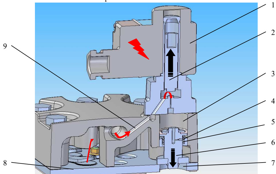
Рисунок 0-1 Принцип работы CR головки
