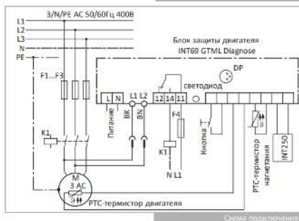
Схема подключения
