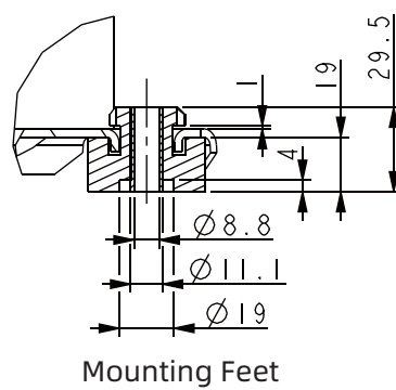
Чертеж виброопоры
