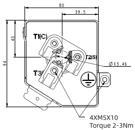
Клеммная коробка
