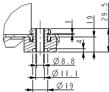
Чертеж вибропоры
