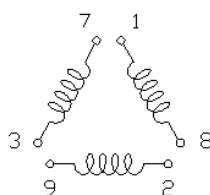
MOTOR WIRINGS
